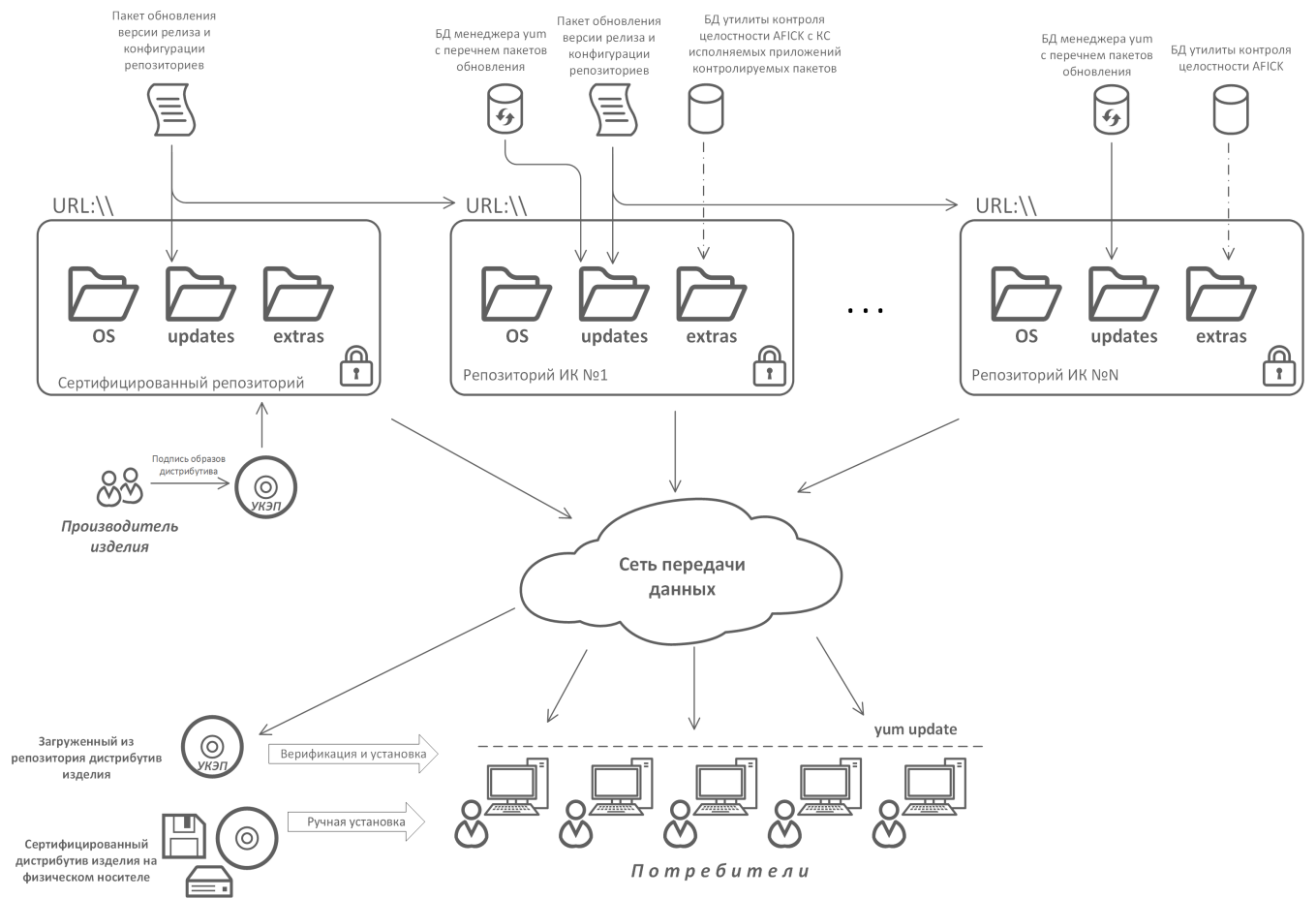
Схема обновления изделия с использованием репозитория
